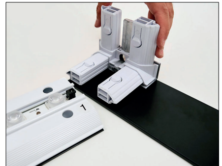
BASE SINISTRA 26x10x0,6 con ANGOLARE Componente IWPLF1200A3 Materiale: pvc e alluminio
