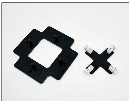
CONNETTORI QUADRATI (superiore ed inferiore) Componenti IWPLF1200V50A / IWPLF1200V50B Materiale: pvc e alluminio
