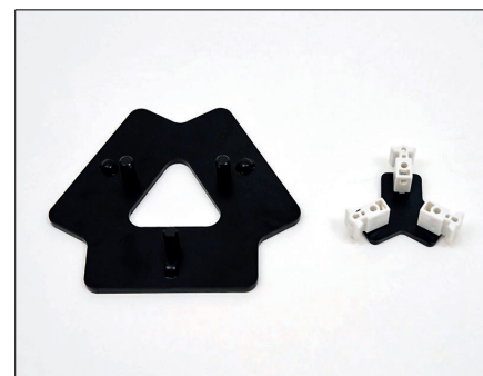
CONNETTORI TRIANGOLARI (superiore ed inferiore) Componenti IWPLF1200V40A / IWPLF1200V40B Materiale: pvc e alluminio
