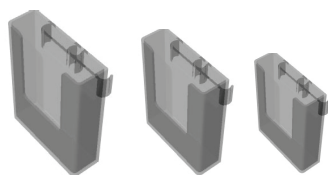
PORTA BROCHURE A6, A5, A4 con clip a C Componente n° 5061 / 5062 / 5063 Materiale: metacrilato Peso: 0,140 Kg, 0,160 Kg, 0,330 Kg
