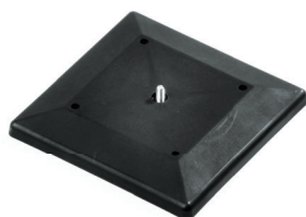
BASE 16x16 cm Componente n° 3066 Materiale: composito alluminio e plastica Peso: 0,160 Kg
