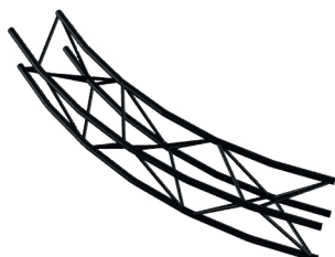
TRALICCIO CURVO 60 cm raggio 70 Componente n° 3075 Materiale: composito alluminio e plastica Peso: 0,570 Kg
